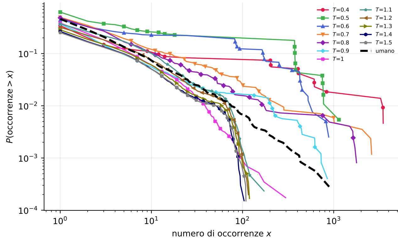
Istogramma cumulativo — Qwen2.5-14B (cfr. [Z] Fig. 6)
