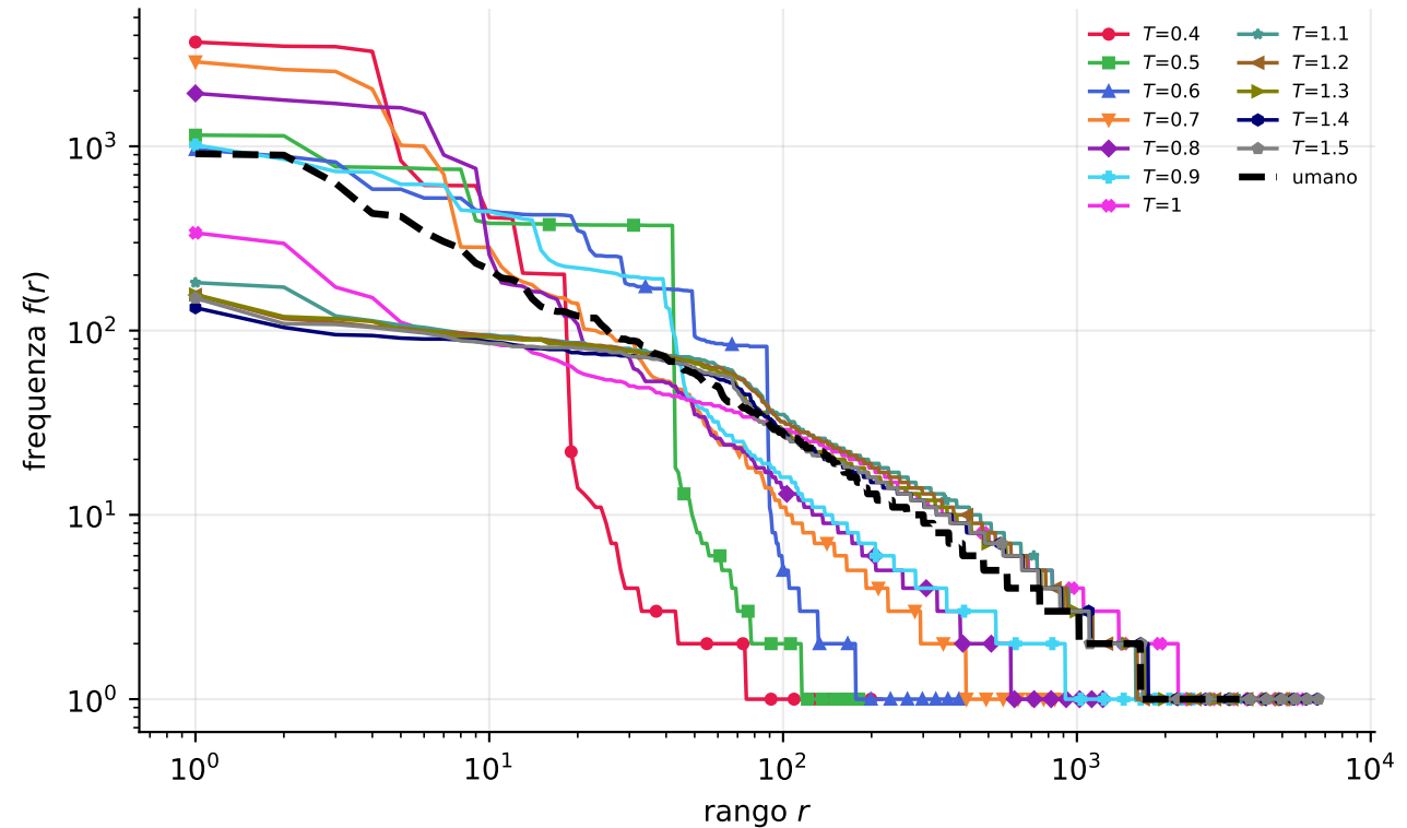
Rango-frequenza — Qwen2.5-14B (cfr. [L] Fig. 2A)
